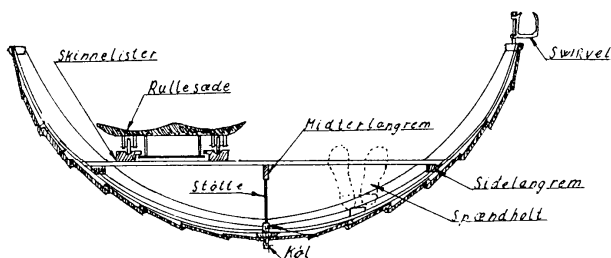
Snit af inrigger.
